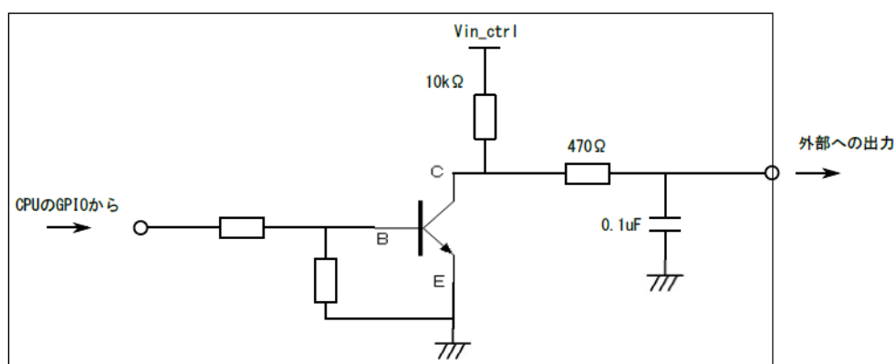
図4.7-2 DO回路図
