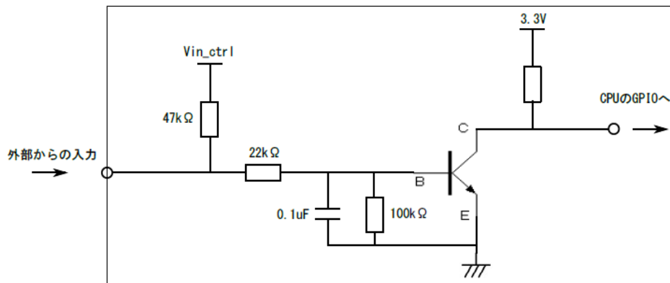
図4.7-1 DI回路図
