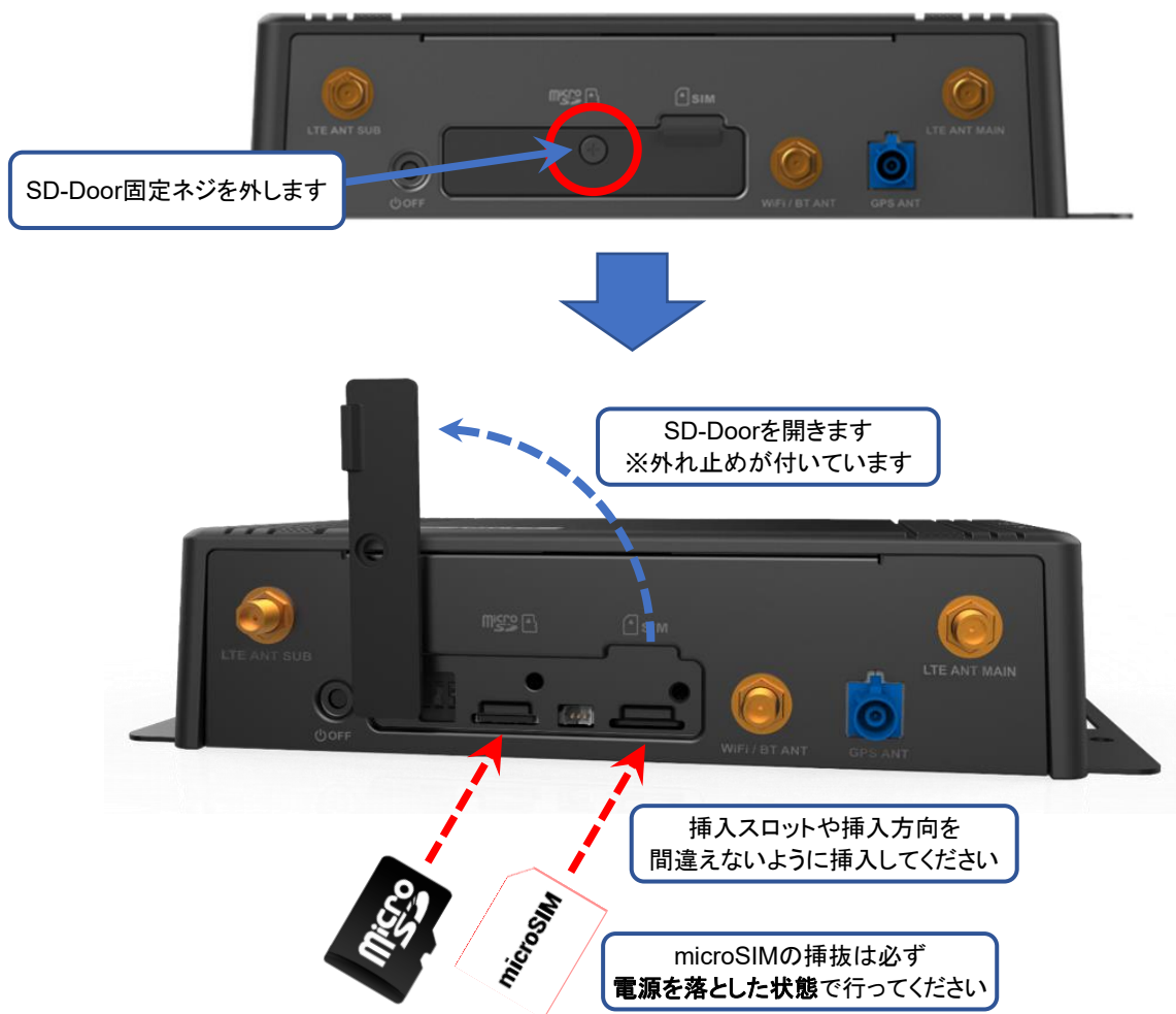
図3.1-1 microSIM および microSDの挿入
